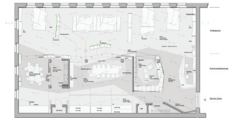
Grundriss
