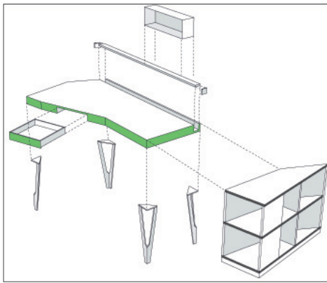
Explosionszeichnung Tisch + Zusatzelemente
